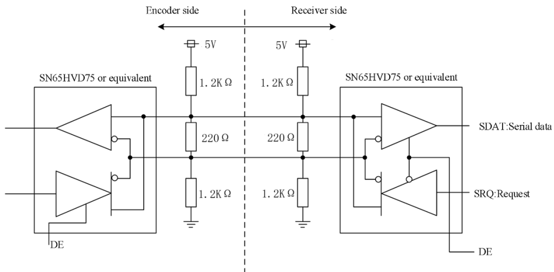
图 4-4-5 发送和接收接口电路示例图
